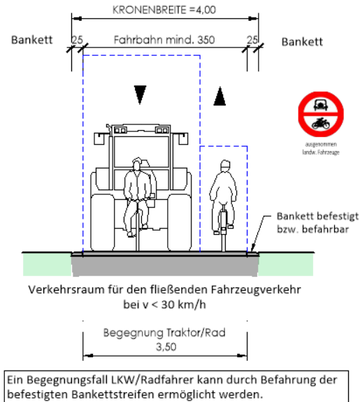
QUERSCHNITT (I) - Abschnitt 1 + 2 M 1: 100 "Radverkehrsführung auf untergeordneten Straßen und Wege" Wirtschaftswege
