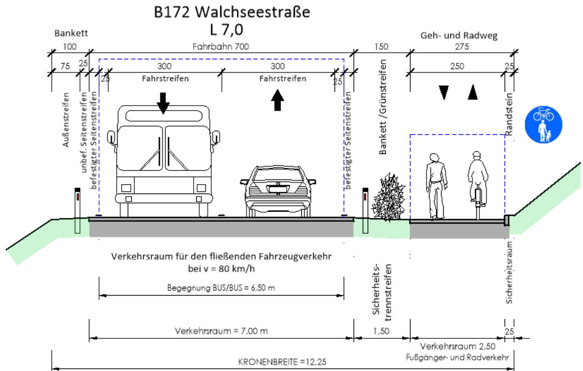
QUERSCHNITT (I) - Abschnitt 1 + 3 M 1: 100 "Radverkehrsführung entlang übergeordneten Straßen außerhalb Ortsgebiet" straßenbegleitender gemischter Geh- und Radweg
