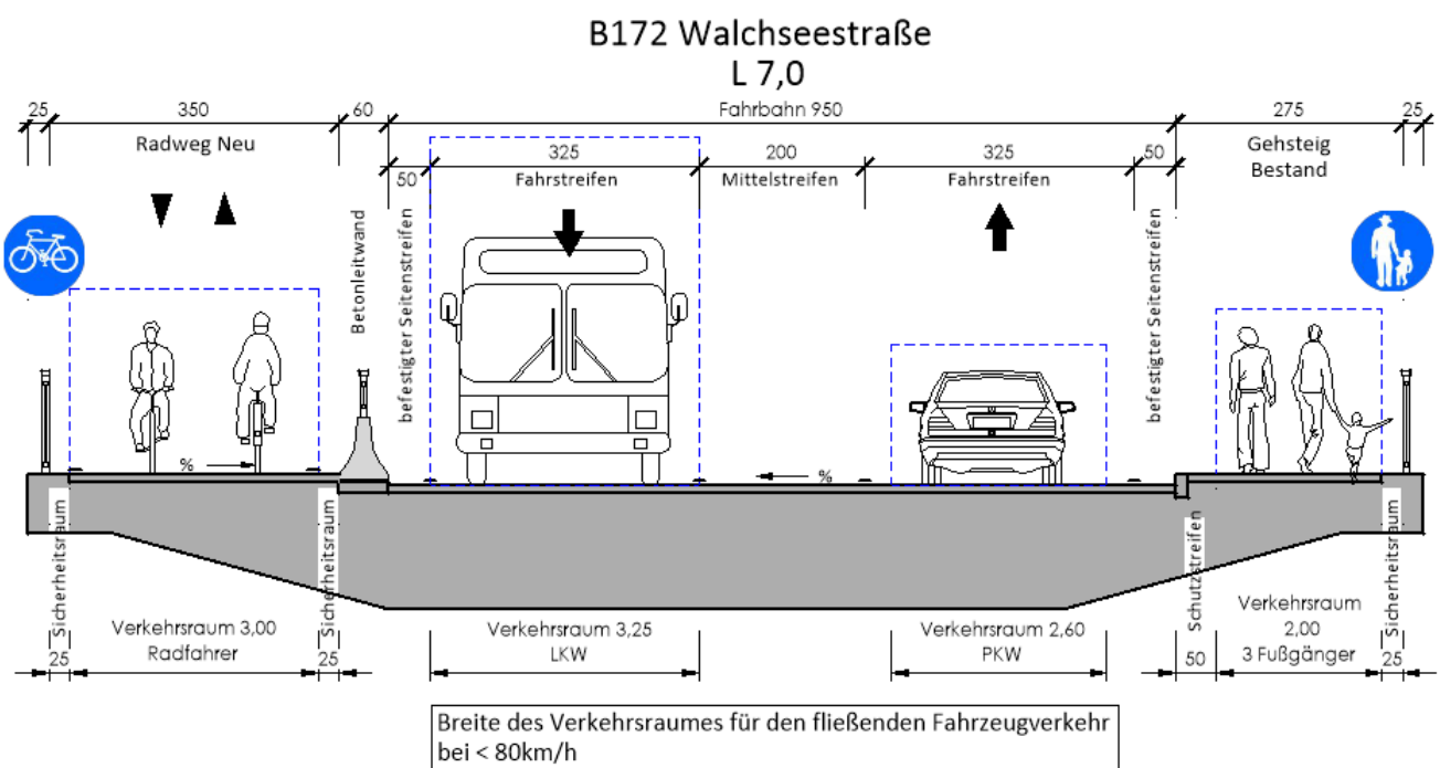
QUERSCHNITT (II) - Abschnitt 3 M 1: 100 "Radverkehrsführung entlang übergeordneten Straßen auf Brückenobjekt" straßenbegleitender Radweg
