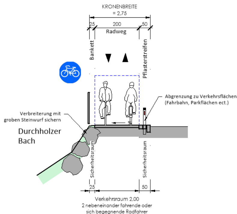
QUERSCHNITT (II) - Abschnitt 2 M 1: 100 "Radverkehrsführung auf Radwege" selbstständig geführter Radweg
