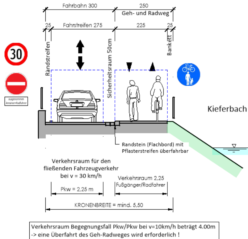
QUERSCHNITT (I) - Abschnitt 1 M 1: 100 "Radverkehrsführung entlang untergeordneten Straßen" gemischter Geh- und Radweg Einfahrt nur für eingeschränkten Kfz-Verkehr und Radfahrer erlauben - unechte Einbahn
