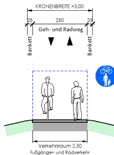
QUERSCHNITT (II) - Abschnitt 2 M 1: 100 "Radverkehrsführung auf selbständig geführten Wege" gemischter Geh- und Radweg
